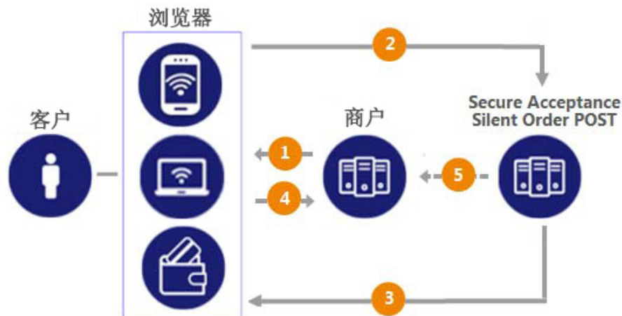
图 1 Secure Acceptance Silent Order POST 交易流程
